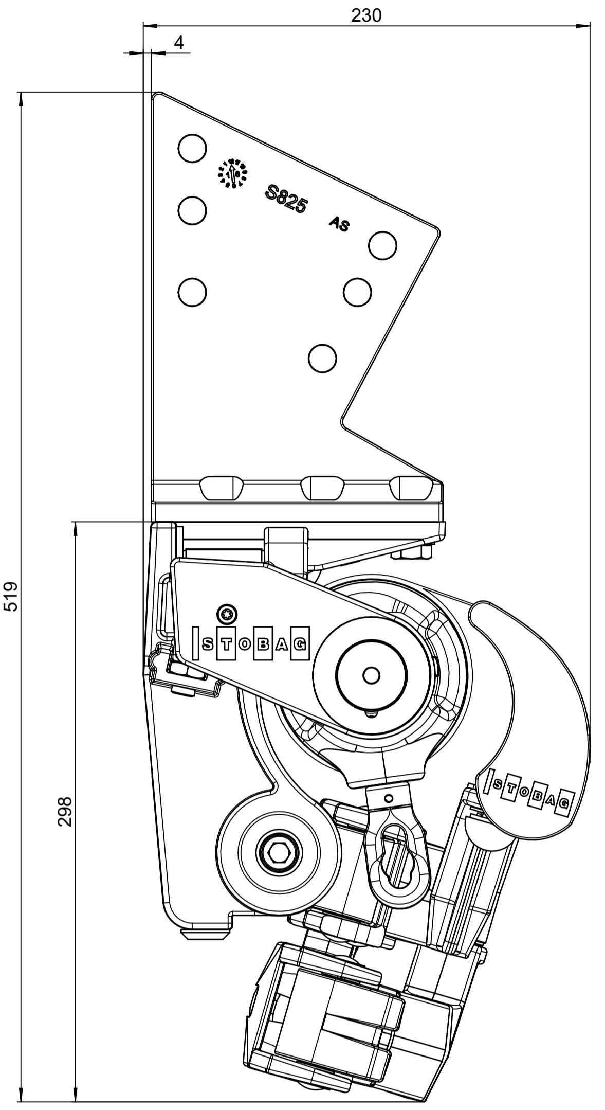
Dachsparrenmontage mit Getriebe
